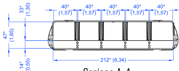
Sezione A-A Section A-A
