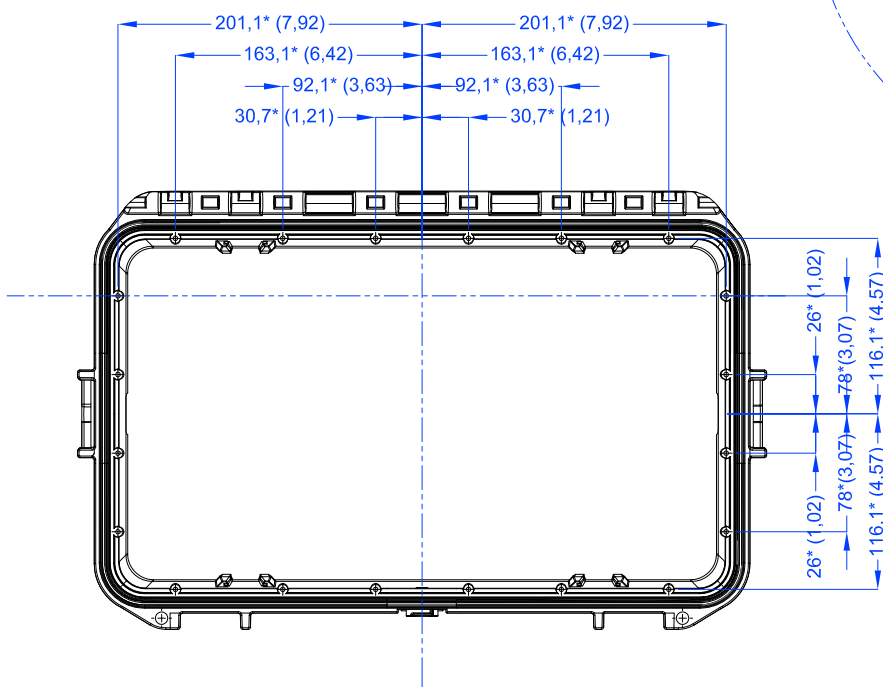
Vista Interna Fondo Bottom Inner View
