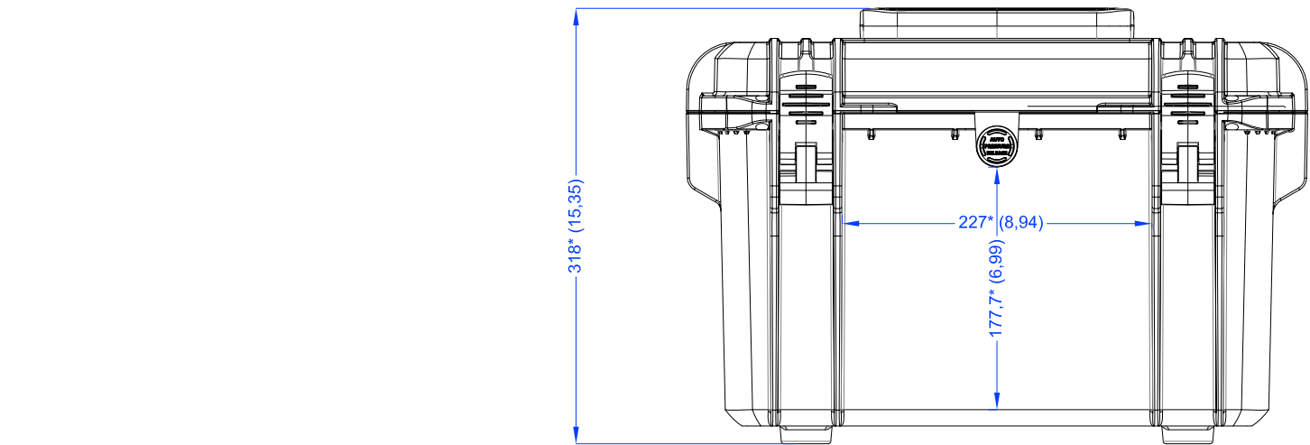
Lato Apertura Opening Side
