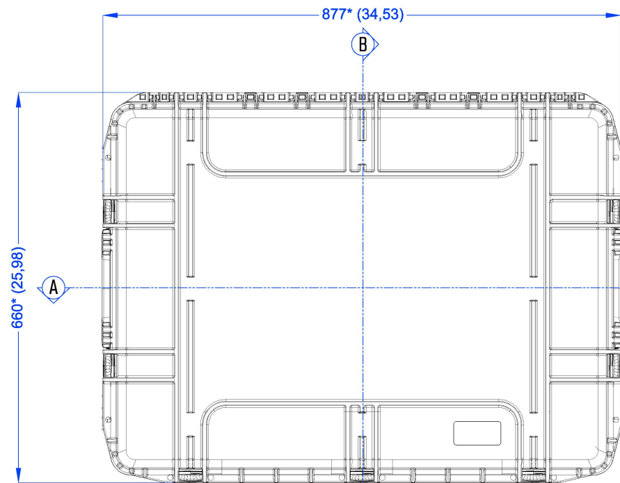
Lato Apertura Opening Side
